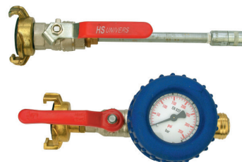
Injektionslanze mit Druckmittler
